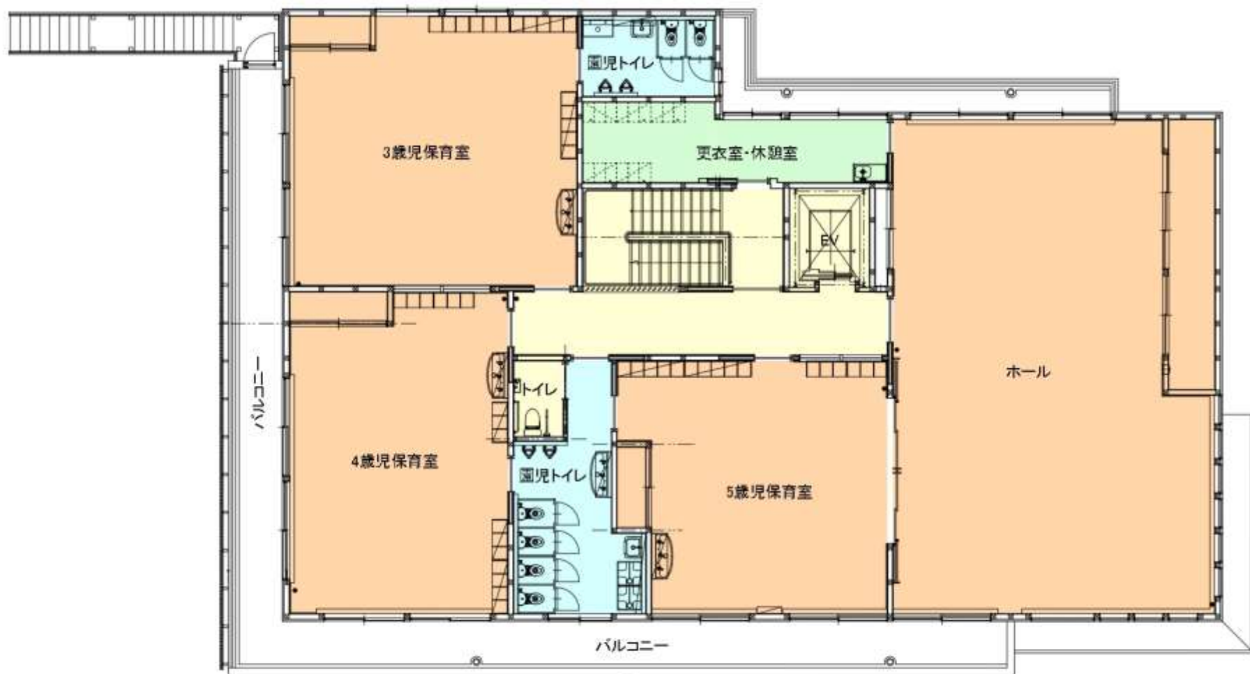
2階平面図
